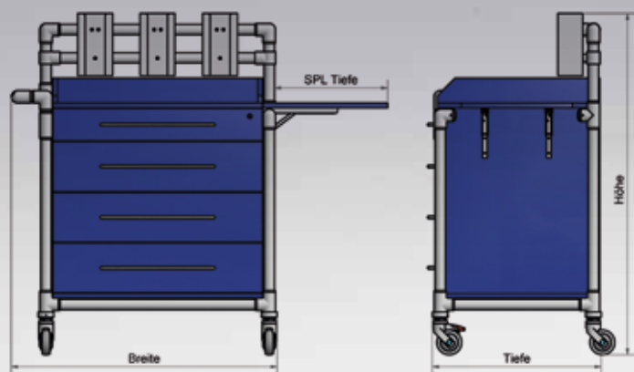
Návrh produktu konstrukčního oddělení po první diskuzi
